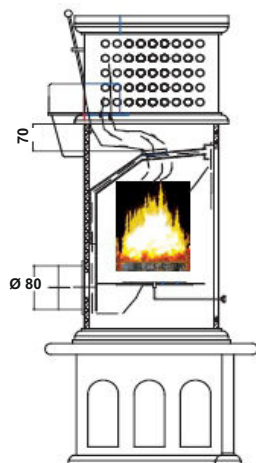
Externer Verbrennungsluftstutzen
