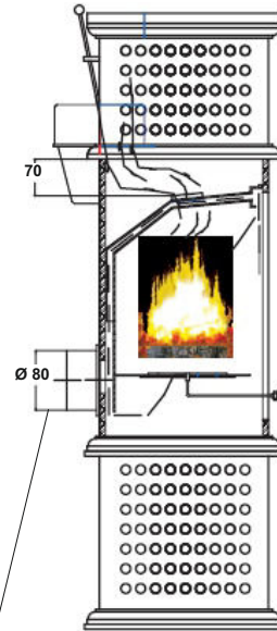
Externer Verbrennungsluftstutzen
