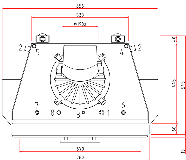
Draufsicht M 1:10
