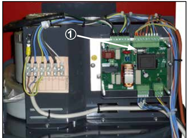
Stuerelektronik AC21 mit der Klemmleiste /1/ - Sicherung 2 A (Typ T2A/1500A 5 x20 mm)
