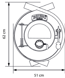
Bruno Mini III
