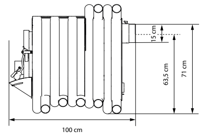
Bruno Pyro IV mit Herdplatte / with hob / avec cuisinière / con piano cottura
