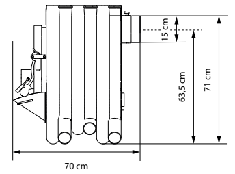
Bruno Pyro II mit Herdplatte / with hob / avec cuisinière / con piano cottura
