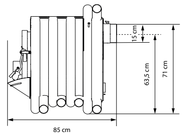
Bruno Pyro III mit Herdplatte / with hob / avec cuisinière / con piano cottura
