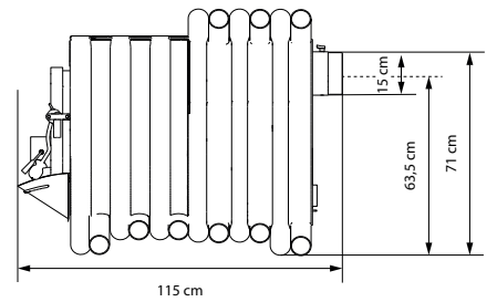
Bruno Pyro V mit Herdplatte / with hob / avec cuisinière / con piano cottura
