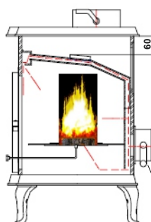
Externer Verbrennungsluftstutzen
